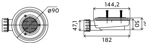
PILETTA DI SCARICO PIATTO DOCCIA
